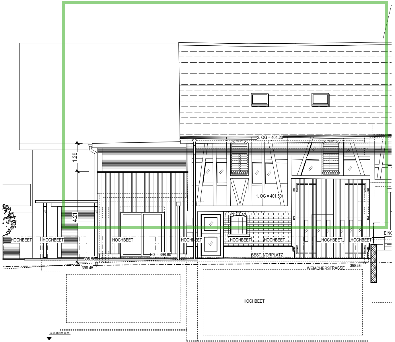
SÜDWESTFASSADE
