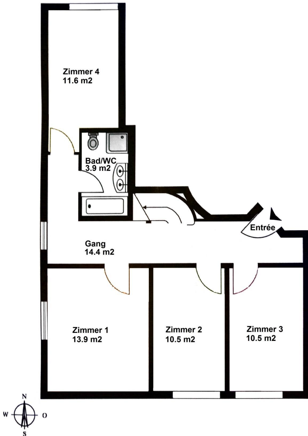
2. Obergeschoss → 5 1/2-Zimmer-Mais.-Wohnung
